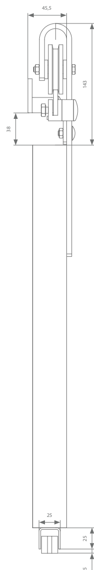
Vloergeleiding optie 1
